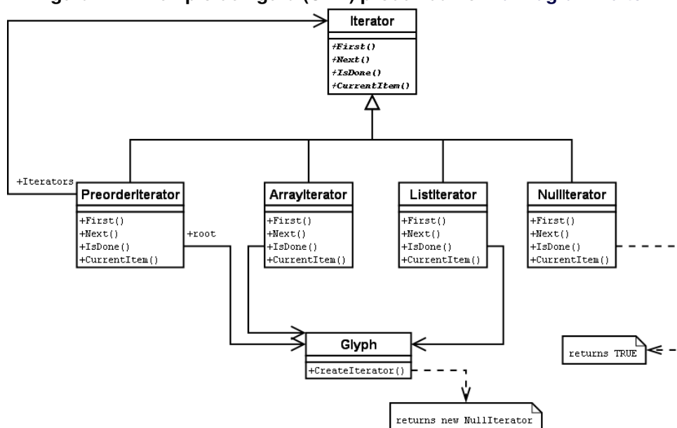
Figura 1 — Exemplo de figura (UML) produzida no Dia Diagram Editor 2
