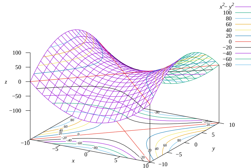
Gráfico 1 — Exemplo de gráfico produzido em gnuplot a partir de arquivo de script a
