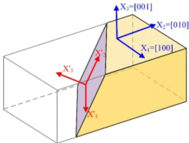
图 2-1 晶体坐标系和样品坐标系示意图
