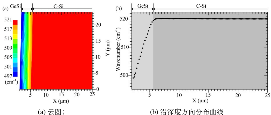
图 2-2 应变硅横截面样品的拉曼类硅峰峰位
