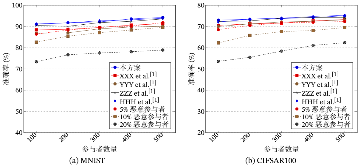
图 2-5 准确度比较
